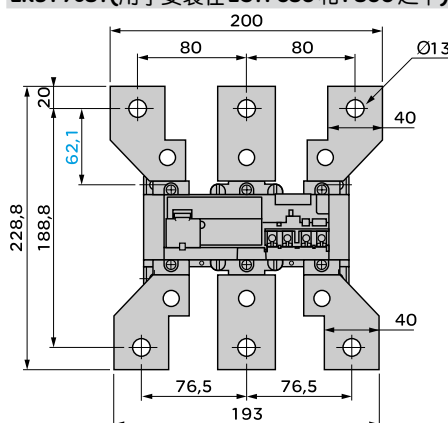
LR9 F781 (用于安装在LC1 F630和F800之下)
