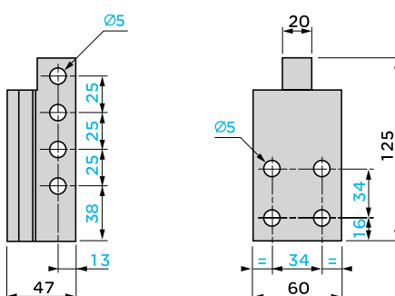
直角连接器LA9 F2100, 用于后部连接(一套6个)
