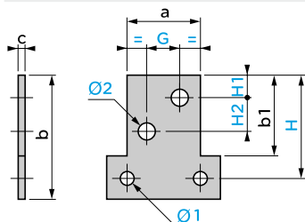
3极星形连接的连接排
