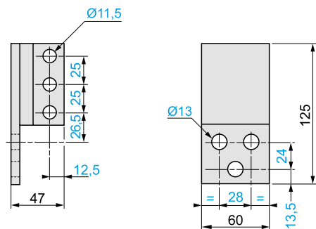
并联接头 (一套4个)
