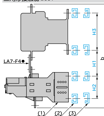
可逆接触器 LC2 F 或星型/ 三角形接触器 LC3 F
