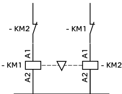
可逆接触器的电气互锁装置，装有： 机械互锁装置 不带集成电气触点
