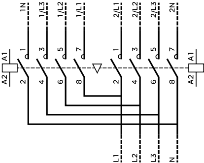
配电用的电源转换接触器组，水平安装
